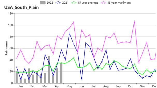
(h). 大平原南部地区降水时间过程线
