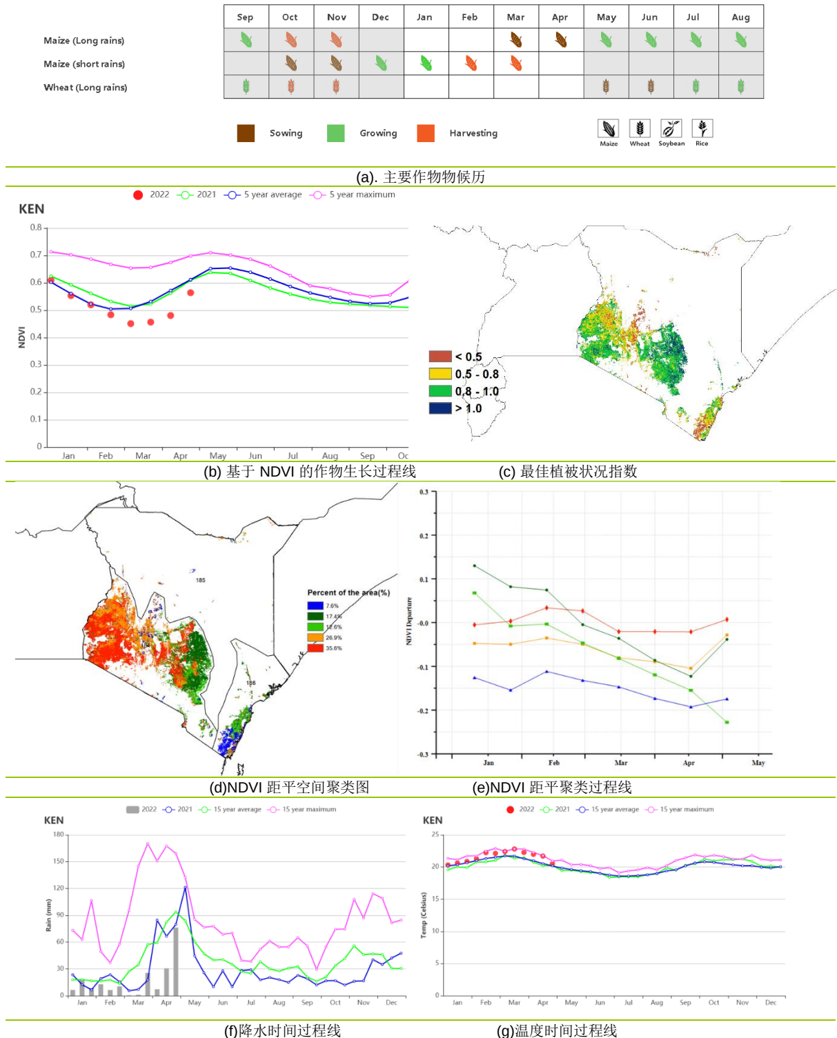
图 3.24 2022 年 1 月-4 月肯尼亚作物长势
