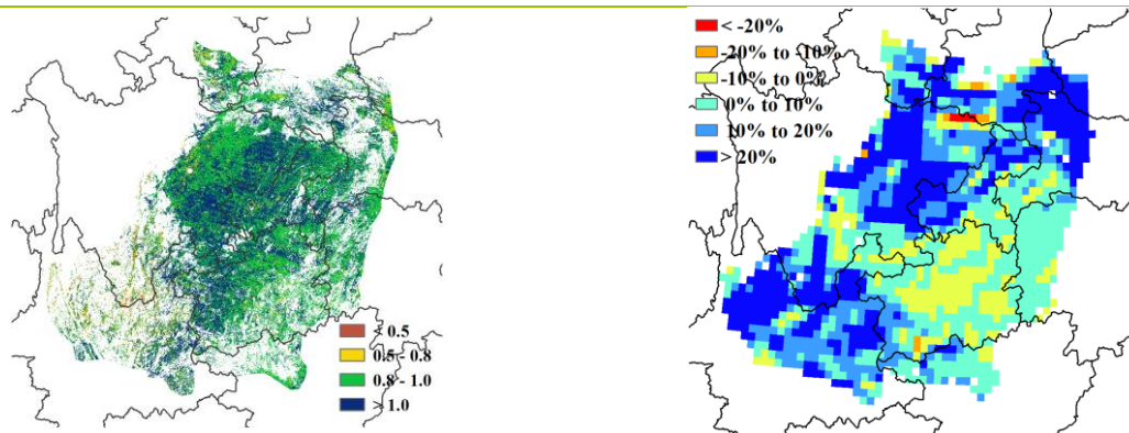
(f) 最佳植被状况指数 (g) 潜在生物量距平
