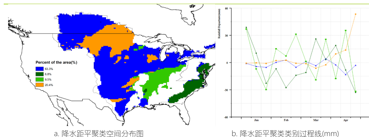
图 2.2 北美农业主产区的农业气象指数与农情指标（2022 年 1 月-4 月）
