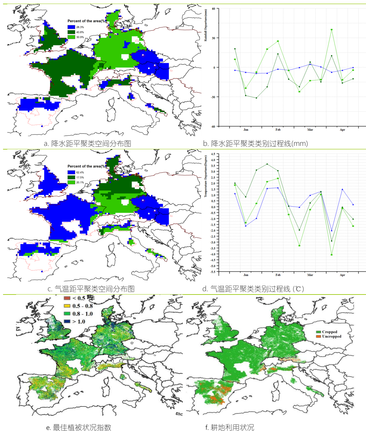
图 2.5 欧洲西部农业主产区的农业气象指数与农情指标 (2022 年 1 月-4 月)
