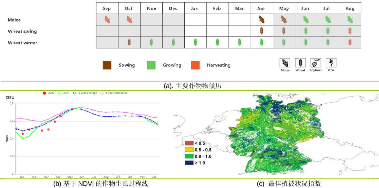
图 3.13 2022 年 1 月-4 月德国作物长势
