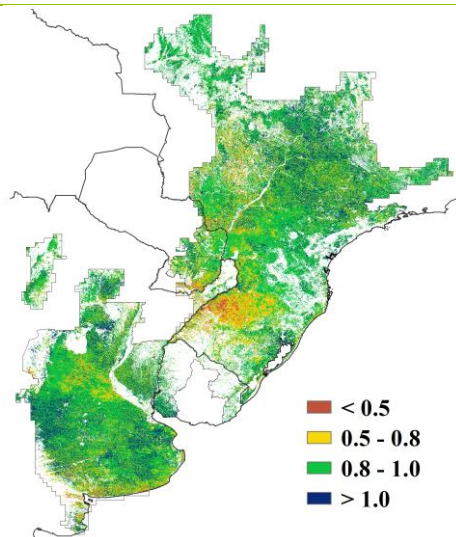
g. 最佳植被状况指数
