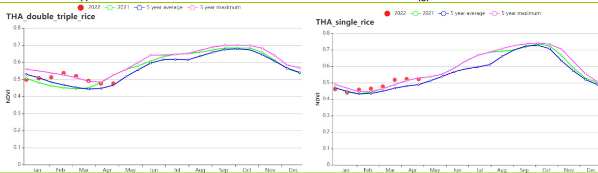
(h) 基于 NDVI 的作物生长过程线 (中部双季和 triple 稻种植区 (左) 和西部、南部山地区域 (右))
