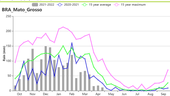
(h) 基于 NDVI 的马托格罗斯及周围地区作物生长过程线 (左) 和时间序列 (旬) 降水过程线 (右)
