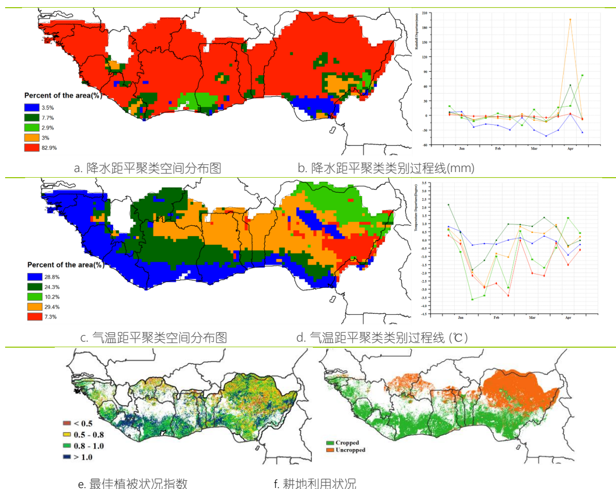
图 2.1 非洲西部农业主产区的农业气象指数与农情指标（2022 年 1 月-4 月）
