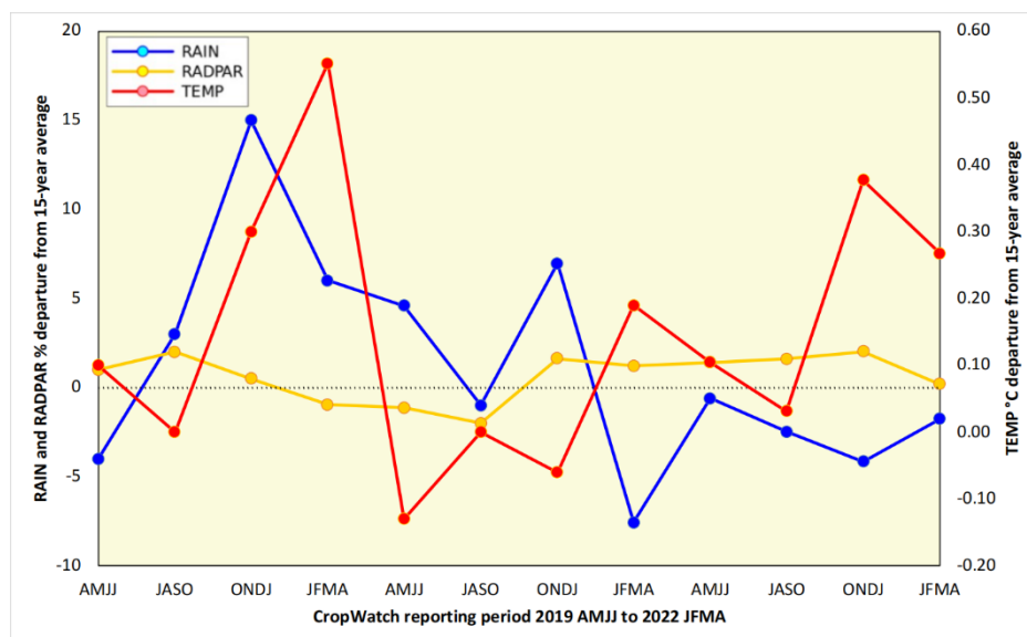
图 1.1 全球分析单元 (MRU) 与过去 15 年同期降水、气温和光合有效辐射距平, 最后一个计算时期涵盖到 2022 年 1 月至 4 月 (65 个全球分析单元算数平均, 未加权重)
