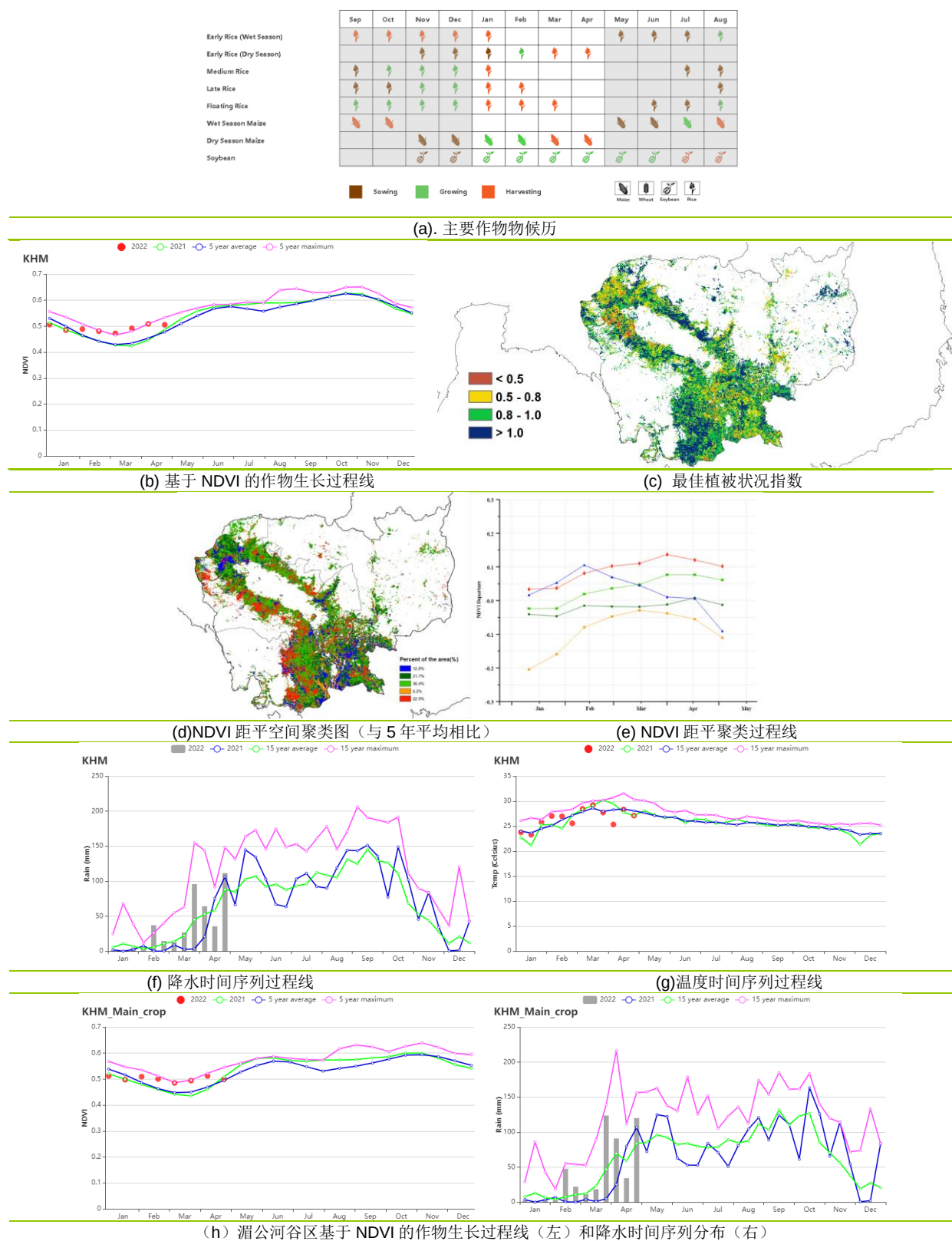
图 3.26 2022 年 1 月-4 月柬埔寨干季作物长势
