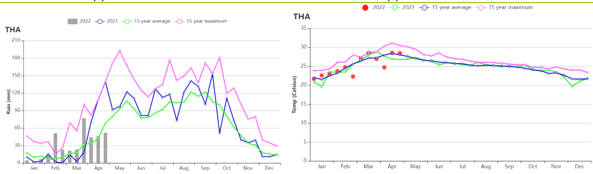
(f) 降水时间序列过程线
