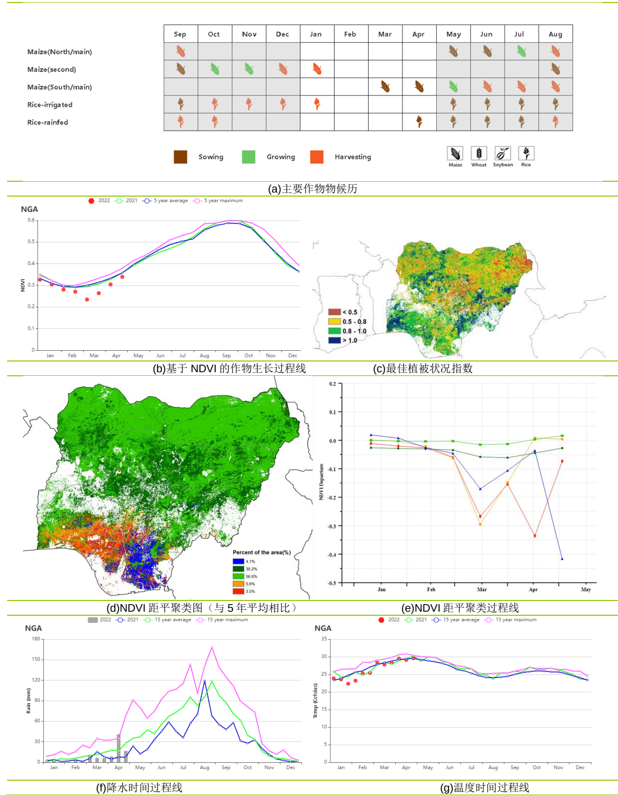
图 3.33 2022 年 1 月-4 月尼日利亚作物长势
