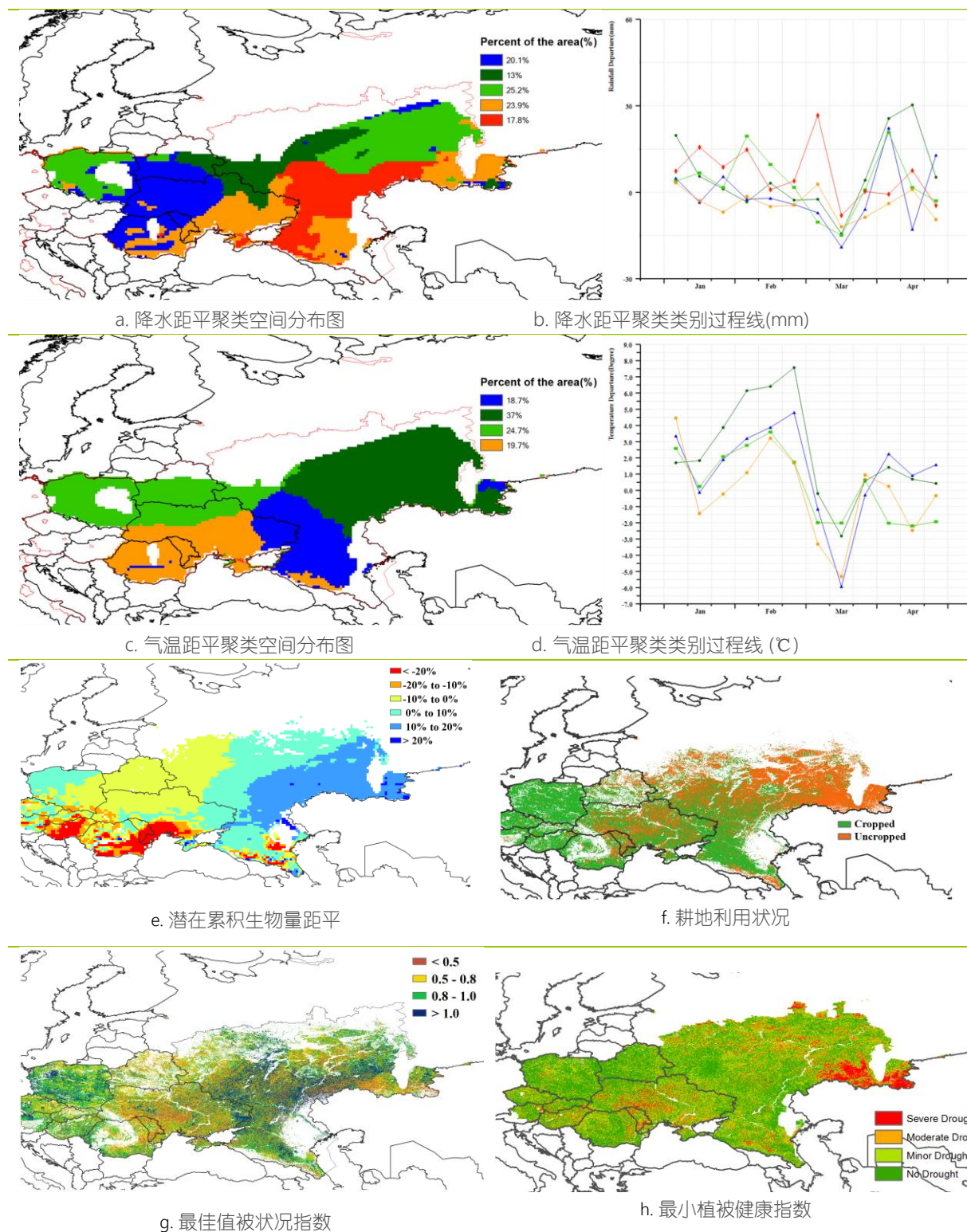
图 2.6 欧洲中部和俄罗斯西部农业主产区的农业气象指数与农情指标（2022 年 1 月-4 月）
