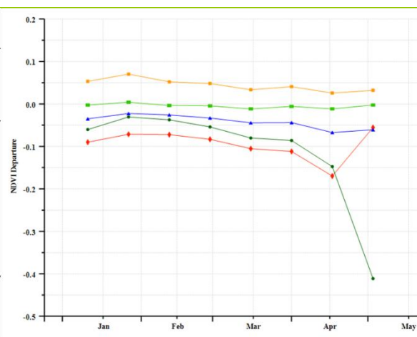
(e) NDVI 距平聚类过程线
