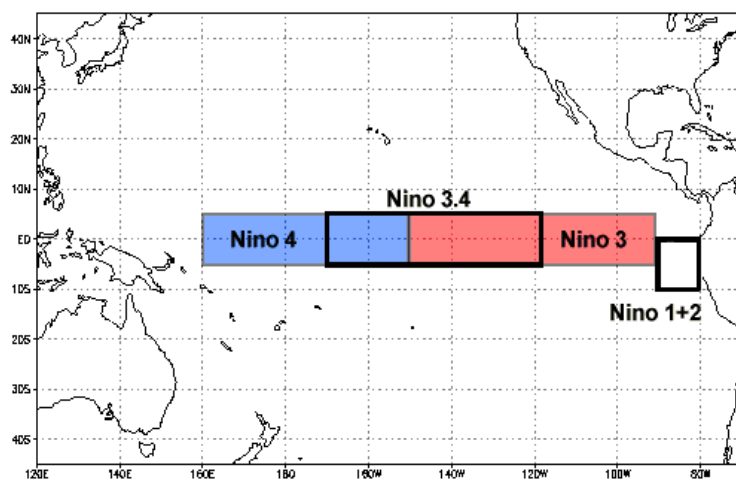
图 5.8 NINO 区域分布图
