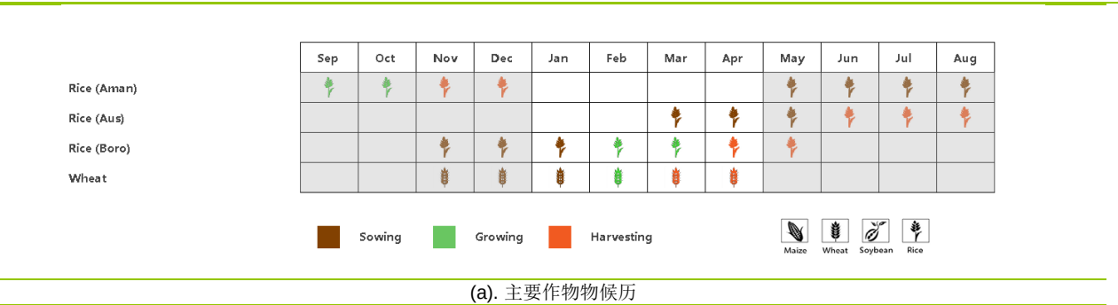
图 3.9 2022 年 1 月-4 月孟加拉国作物长势
