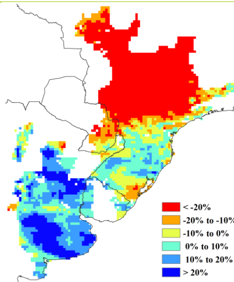
f. 潜在累积生物量距平
