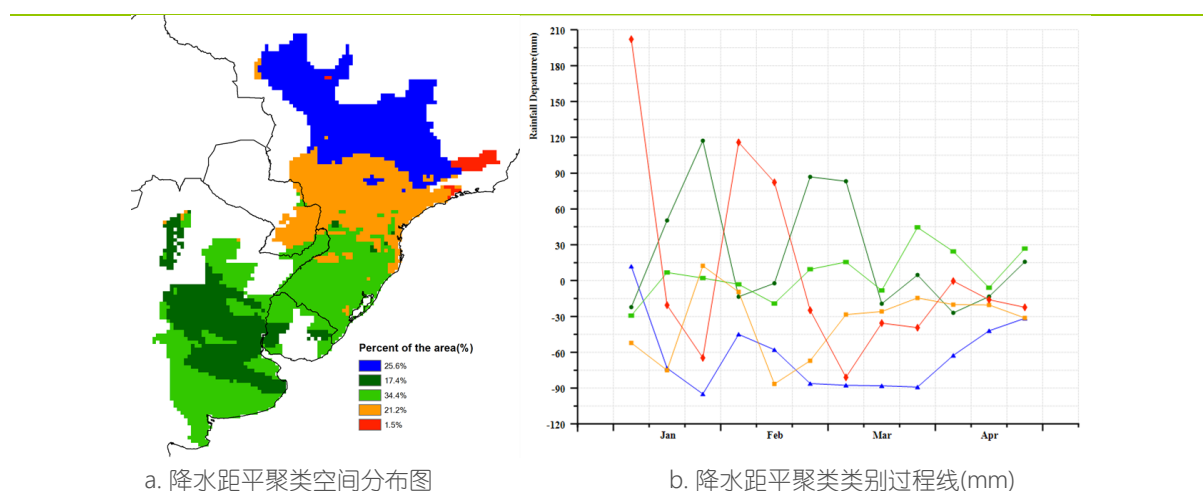
图 2.3 南美洲农业主产区的农业气象指数与农情指标（2022 年 1 月-4 月）
