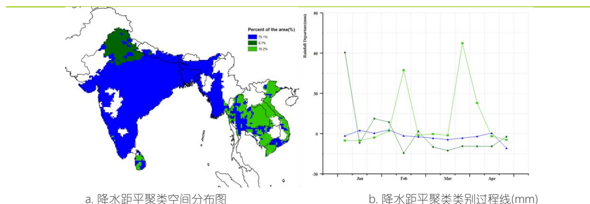
图 2.4 南亚与东南亚农业主产区的农业气象指数与农情指标（2022 年 1 月-4 月）
