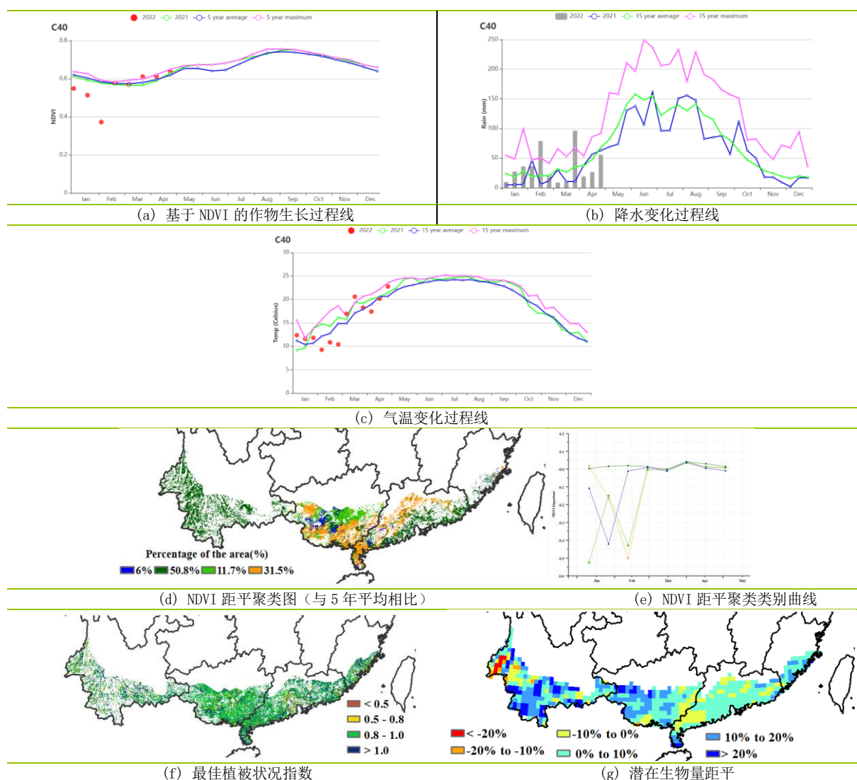
图 4.16 2022 年 1 月-4 月华南区作物长势
