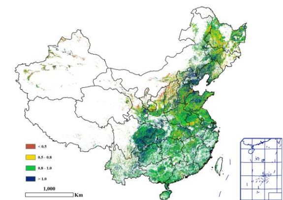
图 4.7 2022 年 1 月-4 月中国最小植被健康状况指数空间分布图
